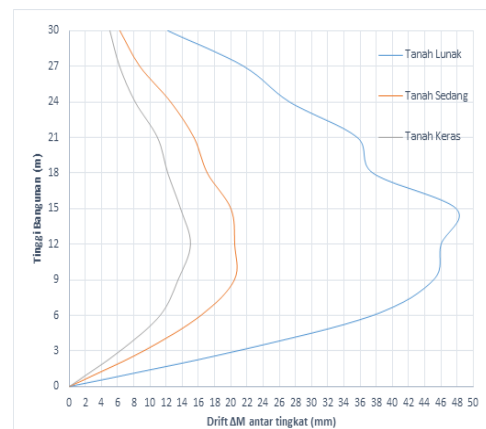
Grafik 3. Perbandingan Drift \Delta M Antar Lantai
