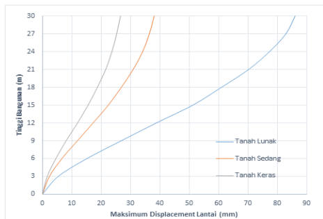
Grafik 1. Perbandingan Maksimum Displacement Lantai
