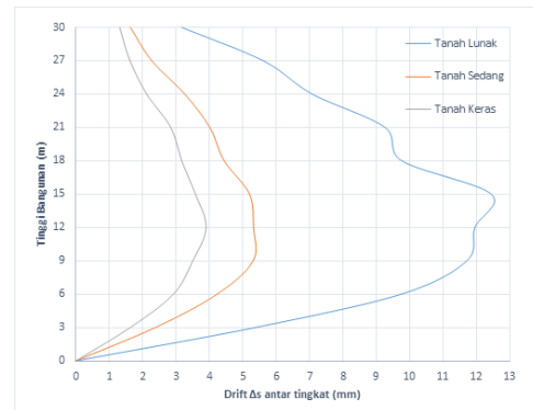
Grafik 2. Perbandingan Drift \Delta s Antar Lantai
