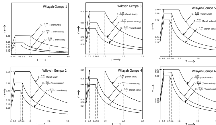
Gambar 3 Respons Spektrum Gempa Rencana
