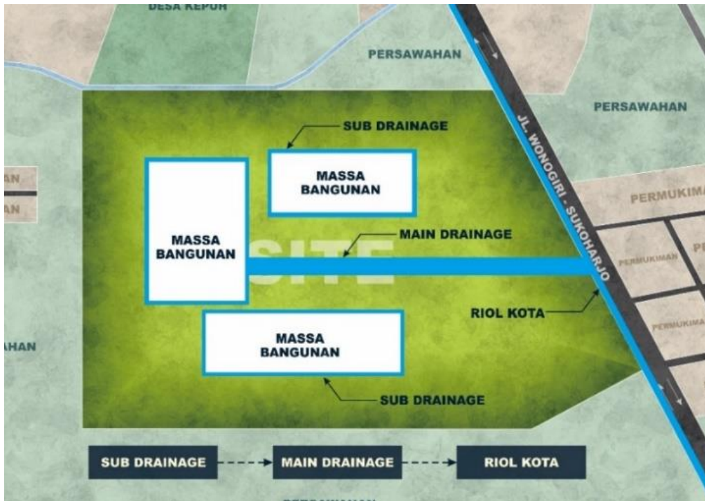
Gambar 17. Sistem Pengolahan Air Hujan Pada Tapak Sumber : Dokumen Pribadi (2023)
