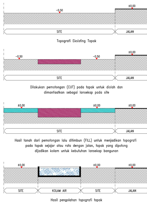
Gambar 4. Topografi Eksisting Tapak Sumber : Dokumen Pribadi (2023)
